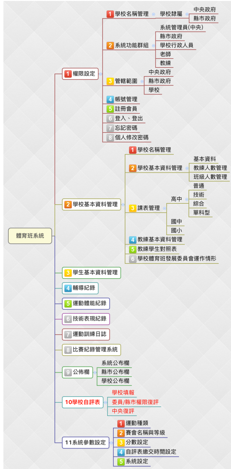
圖 1：系統架構圖
